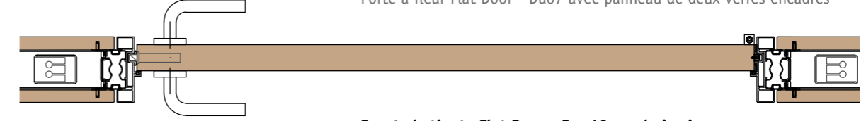
Puerta batiente Flat Door - Duo10 con hoja ciega Porta batente Flat Door - Duo10 com folha cega Hinged door, Flat Door - Duo10 with blank leaf Porte battante Flat Door - Duo10 avec panneau melaminé
