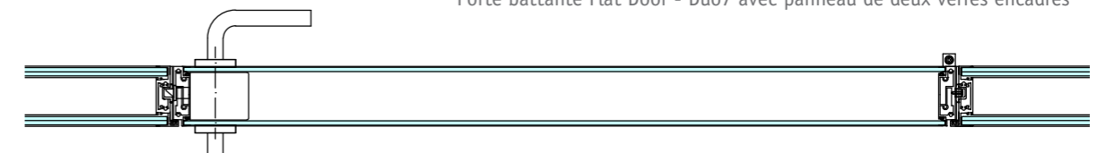
Puerta enrasada Flat Door - Duo7 con hoja de 2 vidrios enmarcados Porta à face Flat Door - Duo7 com folha de 2 vidros encaixilhados Leveled door, Flat Door - Duo7 with double-glazed leaf, alum. frame Porte à fleur Flat Door - Duo7 avec panneau de deux verres encadrés
